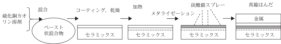
図 4 硫化銅による接合工程 18) .
