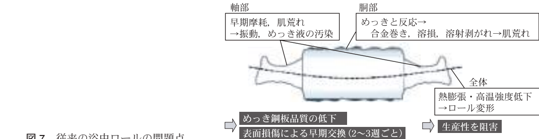
図7 従来の浴中ロールの問題点。
