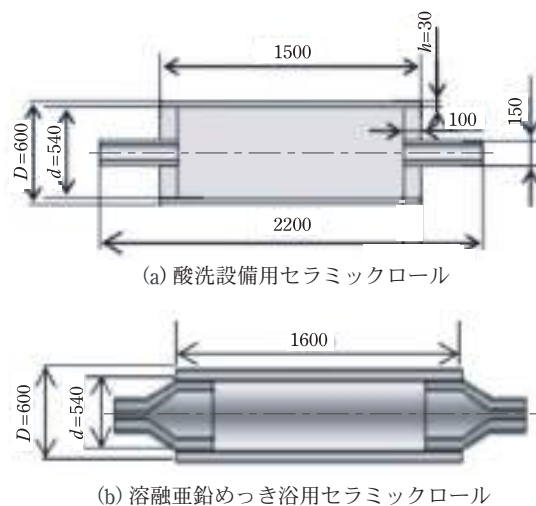
図2 セラミック製スリーブロールの寸法 (mm)。
