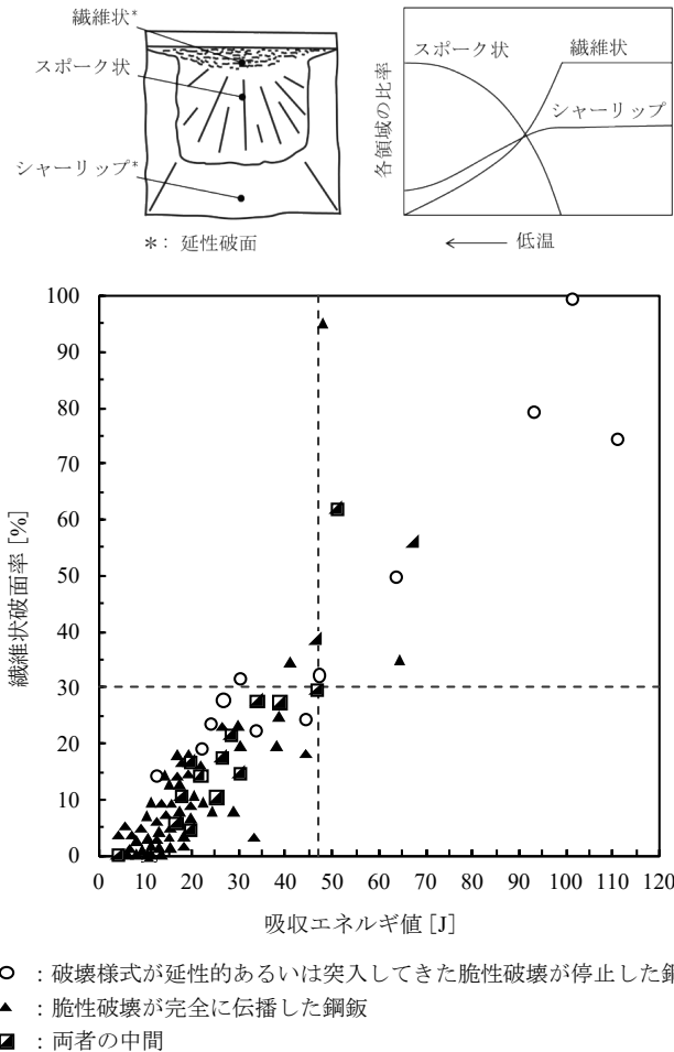
図 1.2 船体用鋼板について損傷時の温度において実施した V ノッチシャルピー衝撃試験での試験片の繊維状破面率と吸収エネルギー値の関係 3), 4)
